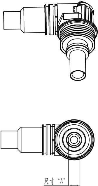
弯头主体
